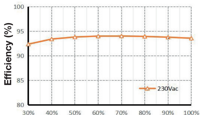
Eficiencia / Efficiency / Efficacité
