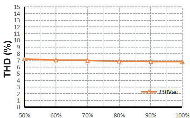
Factor total armónico / Total harmonic factor / Facteur harmonique total (THD)
