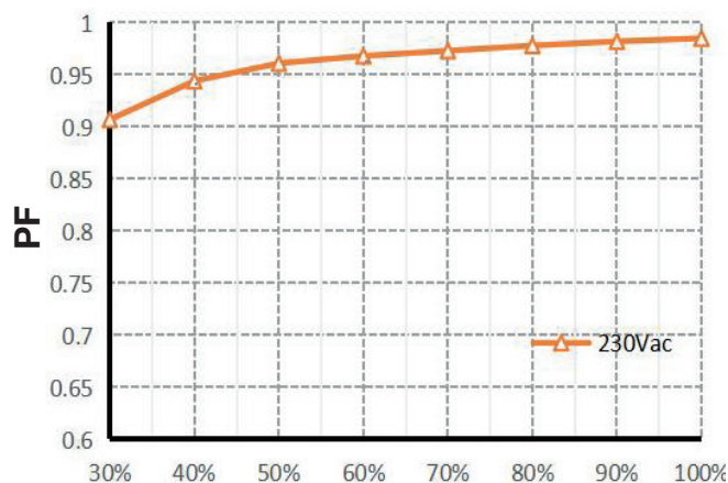
Factor de potencia / Power factor / Facteur de puissance
